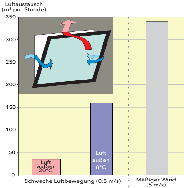
Luftaustausch an einem gekippten Fenster durch Thermik und Windeinfluss.
