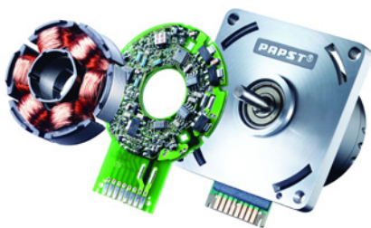
Ein Lüftermotor auf dem Stand der Technik: Die Elektronik sorgt für einen ruhigeren Lauf, bessere Regelbarkeit und einen deutlich höheren Wirkungsgrad.
